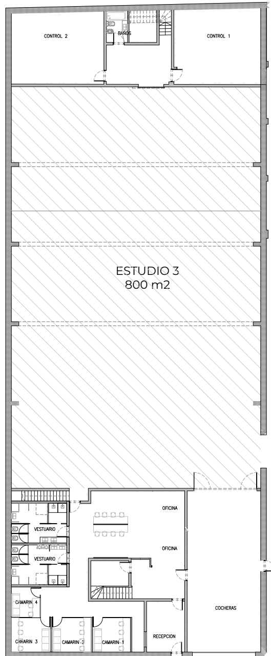
PLANTA BAJA
